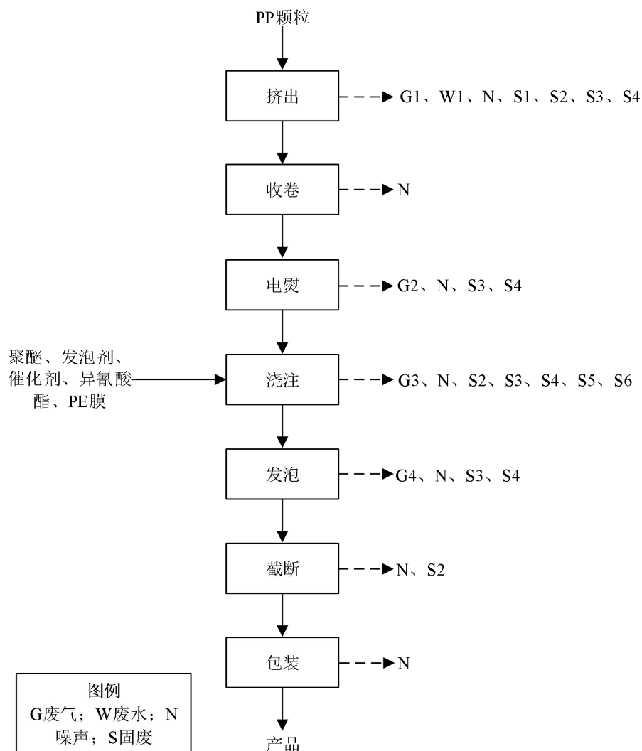
图 2-2 项目工艺流程及排污节点图
