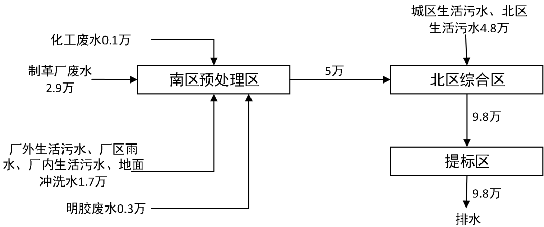
图 4-1 无极县县域污水实际处理量及处理流程图
