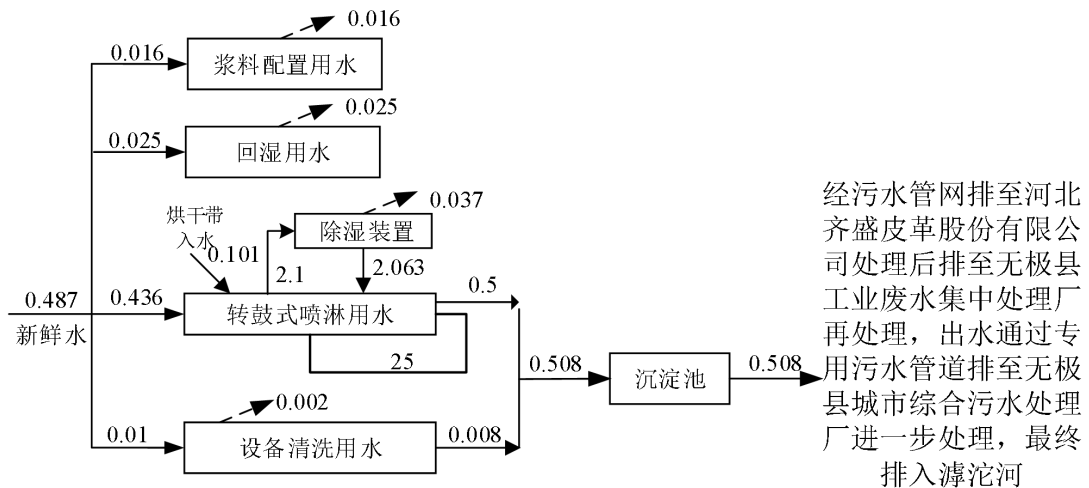
图 2-1 本项目给排水平衡图 (m 3 /d)
