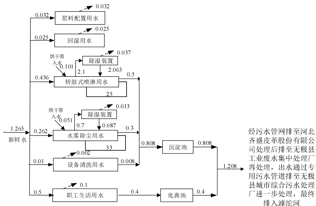
图 2-4 本项目实施后全厂给排水平衡图 (m³/d)
