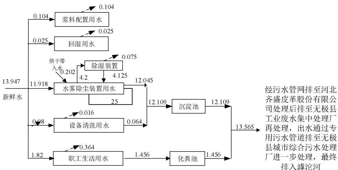
图 2-4 改建项目实施后全厂区给排水平衡图 (m³/d)
