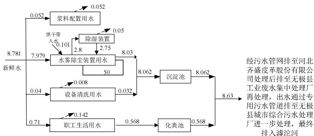
图 2-3 在建项目东厂区给排水平衡图 (m³/d)
