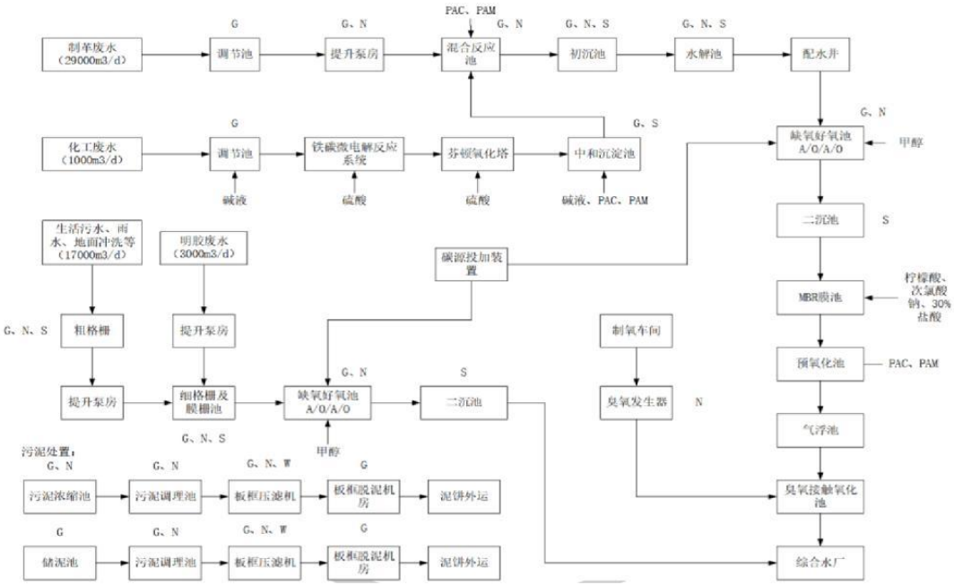
图4-2 南区预处理区—无极县工业废水集中处理厂处理工艺
