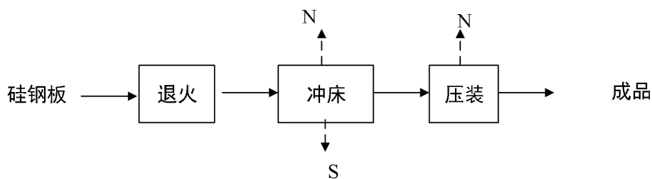
图 2-3 现有工程生产工艺流程及产污环节图
