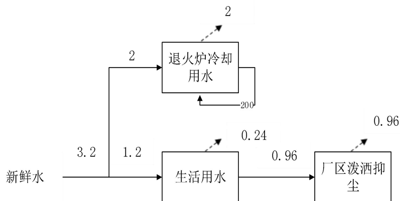
图 2-1 扩建后全厂水平衡图 单位： \text{m}^3/\text{d}
