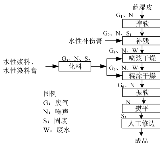
图 2-5 生产工艺及产排污节点图
