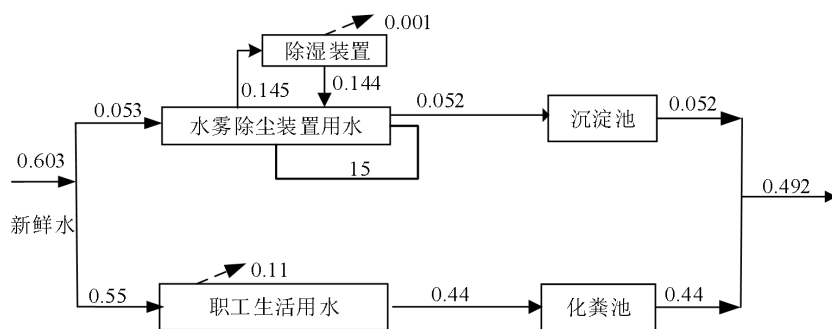
图 2-2 现有工程给排水平衡图 (m³/d)
