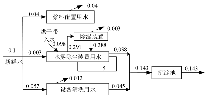
图 2-2 现有工程给排水平衡图 (m³/d)
