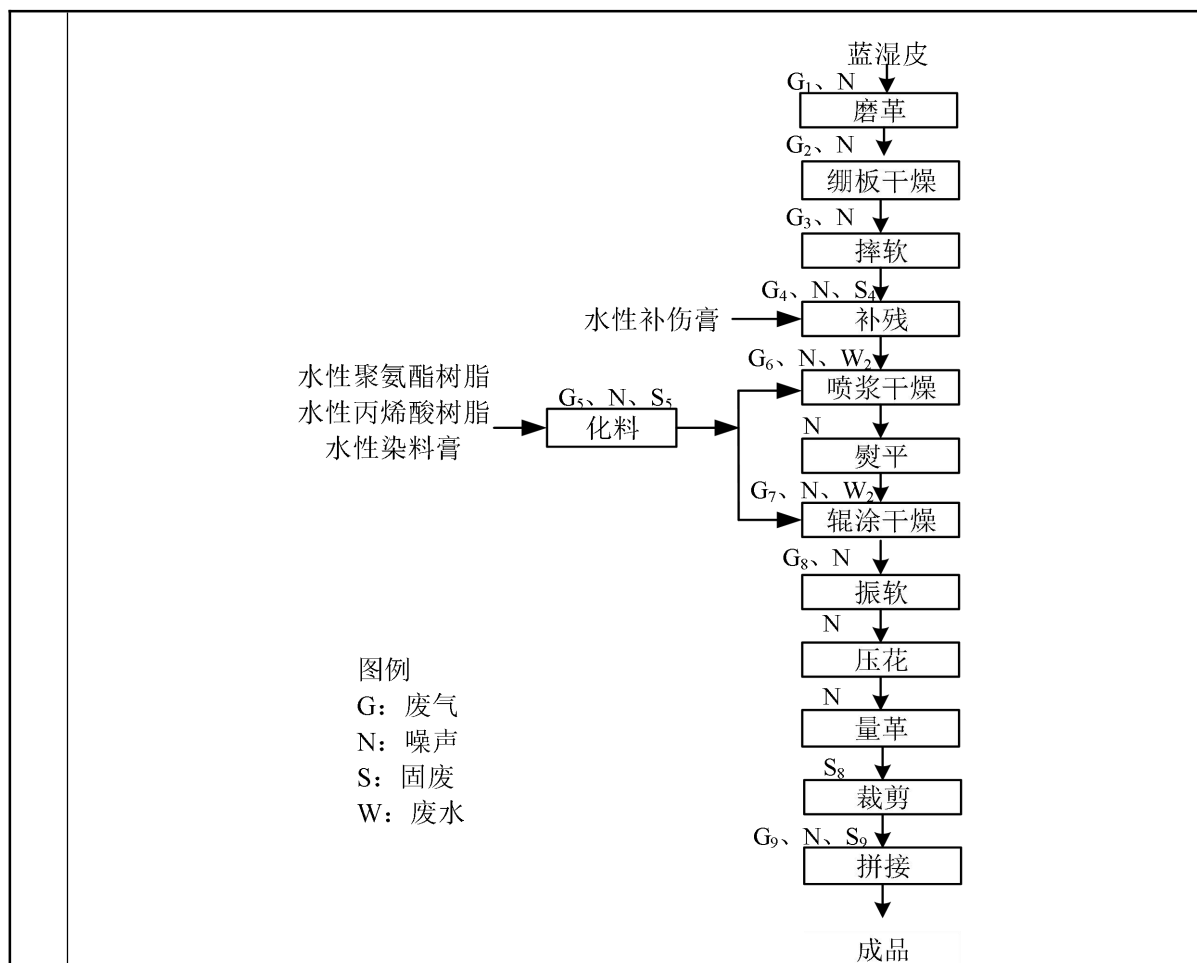
图 2-2 生产工艺及产排污节点图
