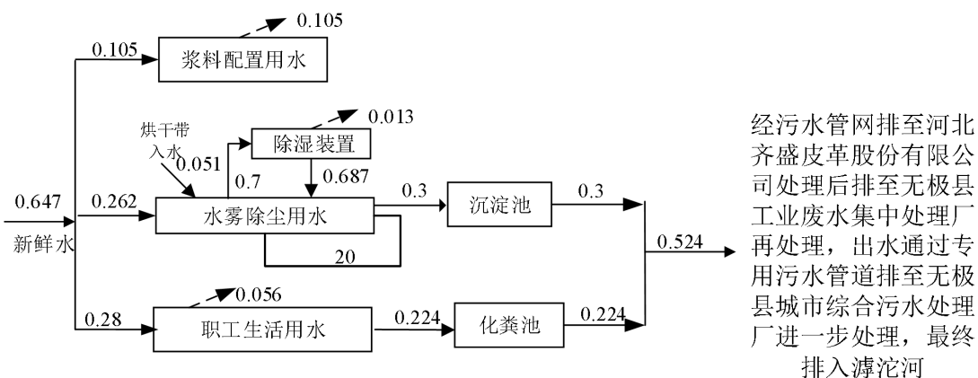
图 2-2 现有工程给排水平衡图 (m³/d)
