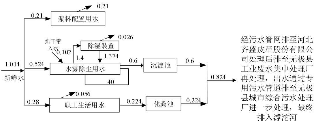
图 2-3 本项目实施后全厂给排水平衡图 (m³/d)
