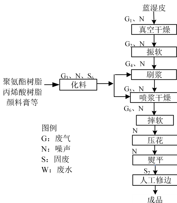
图 2-4 生产工艺及产排污节点图
